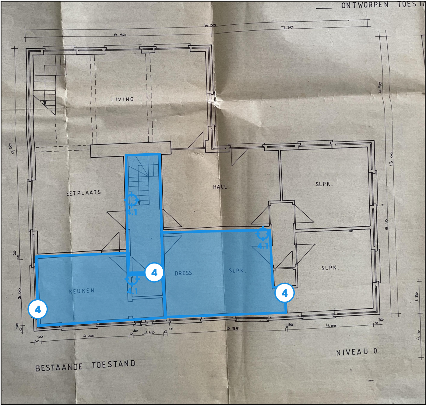
Legende van plan 1.6: grondplan gelijkvloers
